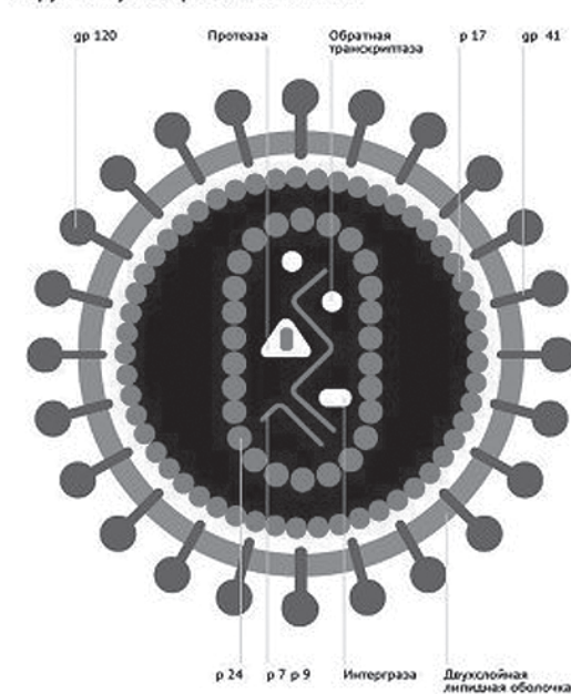
Вирус иммунодефицита в сечении
